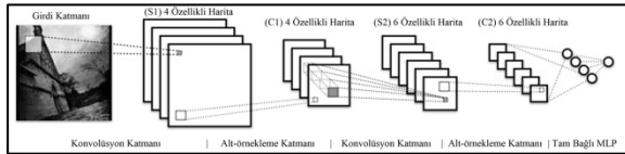
Şekil 3. LeNet ağına mimarisi.
